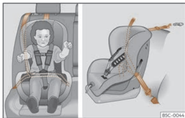
Fig. 38 En los asientos traseros: montaje del asiento para niños.
