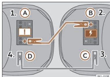
Fig. 186 Esquema de conexión de los cables de emergencia.
