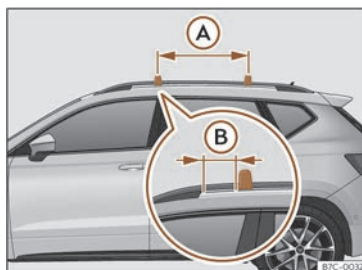
Fig. 174 Puntos de fijación de las barras transversales para el portaequipajes del techo.
