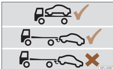
Fig. 187 Transportar con una grúa: vehículos con cambio automático y tracción delantera.
