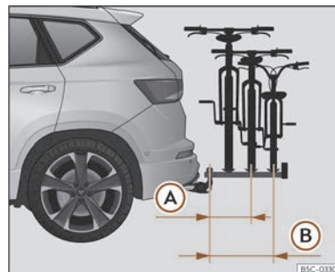
Fig. 178 Representación esquemática del voladizo máximo de la carga en un portabicicletas para dos o tres bicicletas.
