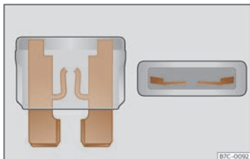
Fig. 196 Representación de un fusible fundido.
