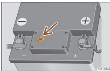
Fig. 207 Mirilla en la parte superior de la batería de 12 voltios (representación esquemática).
