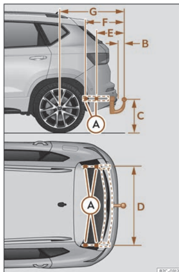
Fig. 179 Cotas y puntos de fijación para el montaje posterior de un dispositivo de remolque.
